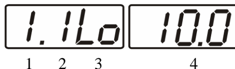
Рисунок 6.12 Поле настройки порогов 1 – параметр (1- температура, 2- влажность) 2 – номер порога (1, 2) 3 – вид порога (Lo – нижний, uP - верхний) 4 – значение порога
